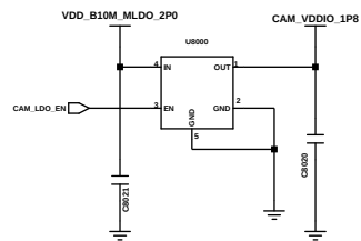
CAM_VDDIO
